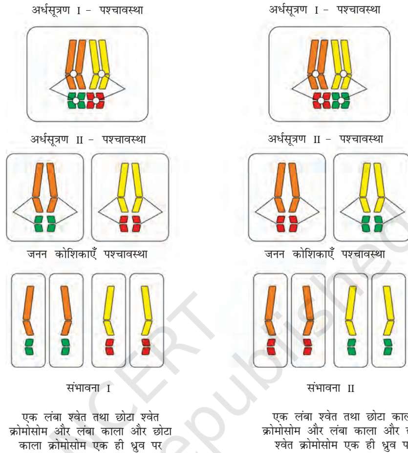
चित्र 4.9 क्रोमोसोमों का स्वतंत्र संव्यूहन
