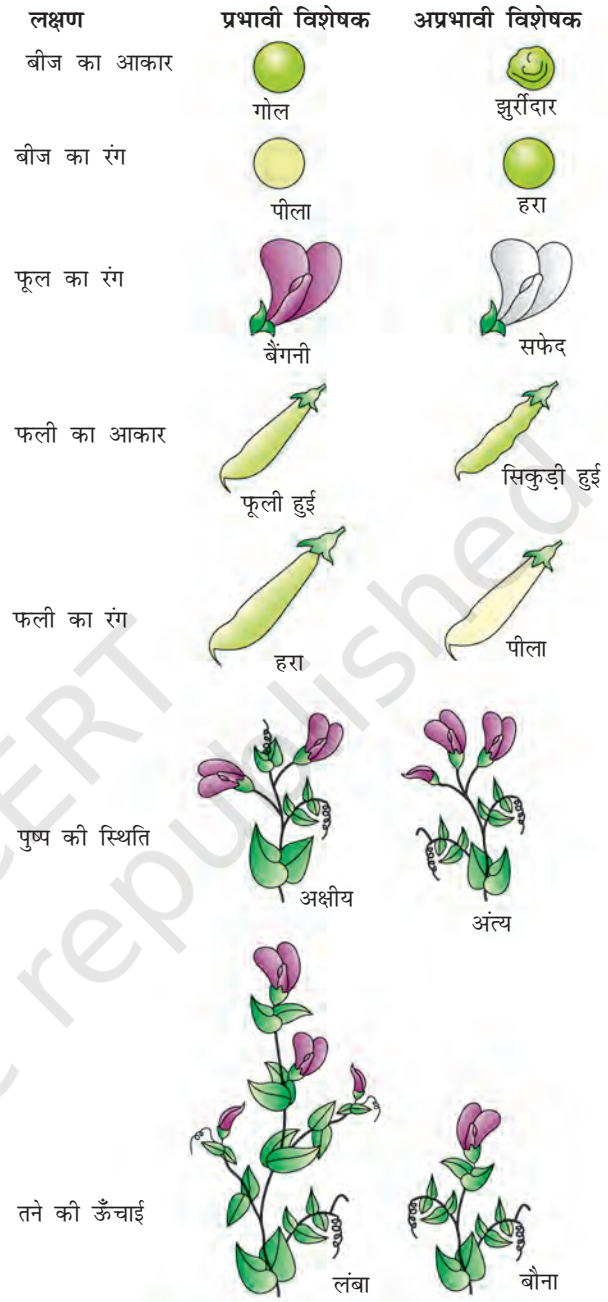
चित्र 4.1 मेंडल द्वारा अध्ययन किए गए मटर के पौधे के विपर्यास विशेषकों के सात जोड़े।
